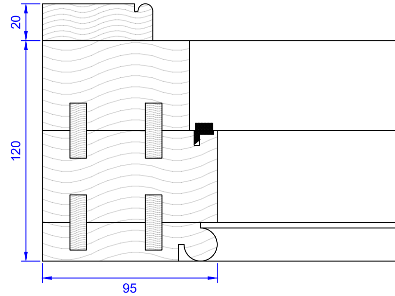
Jamb Section
