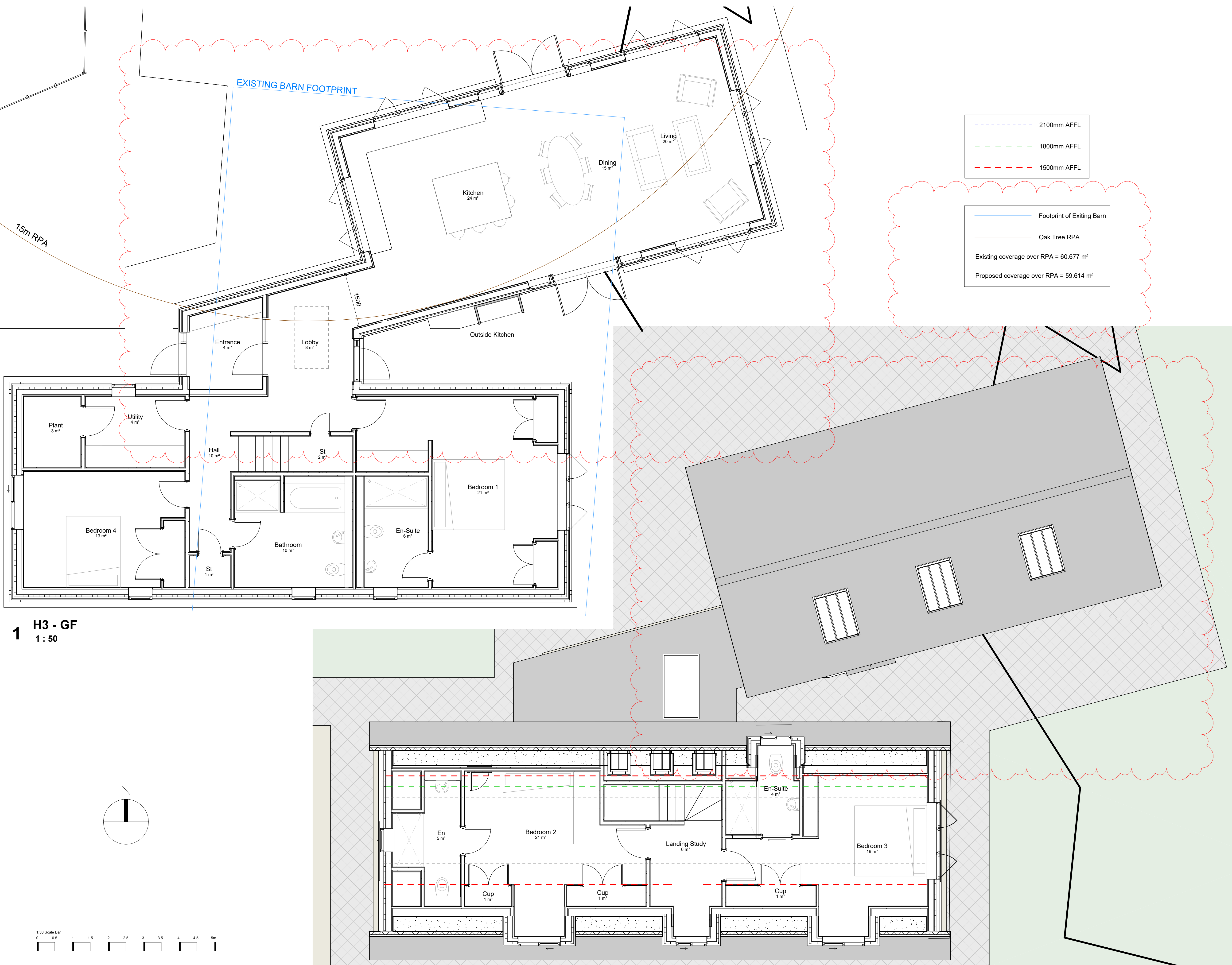
2 H3-FF 1 : 50
