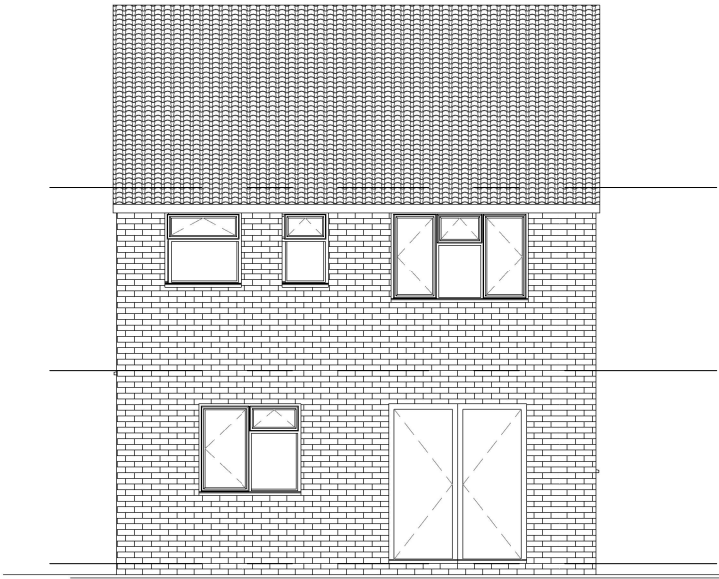
Elevation 'B' 1 : 100
