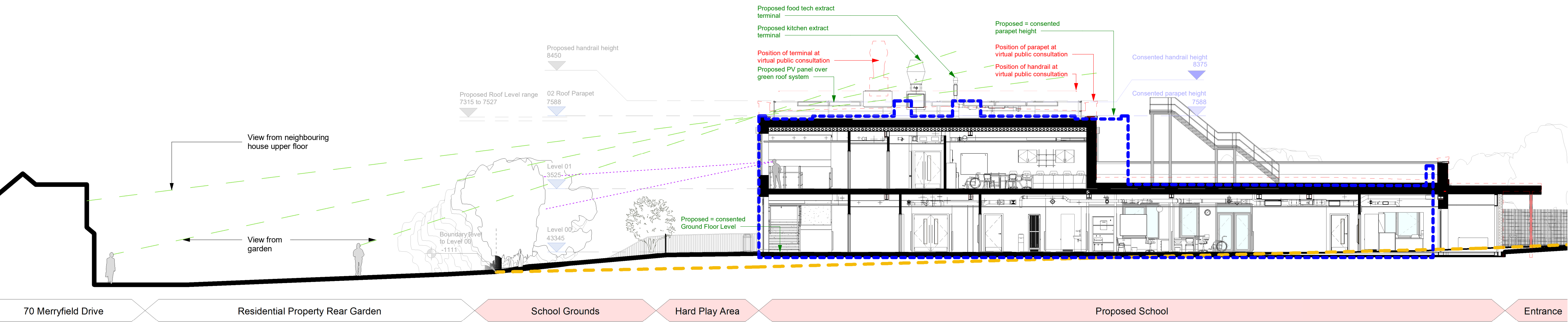
1 Site Section AA 1 : 125
