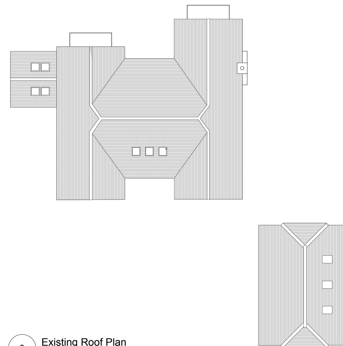
3 Existing Roof Plan Scale: 1:200
