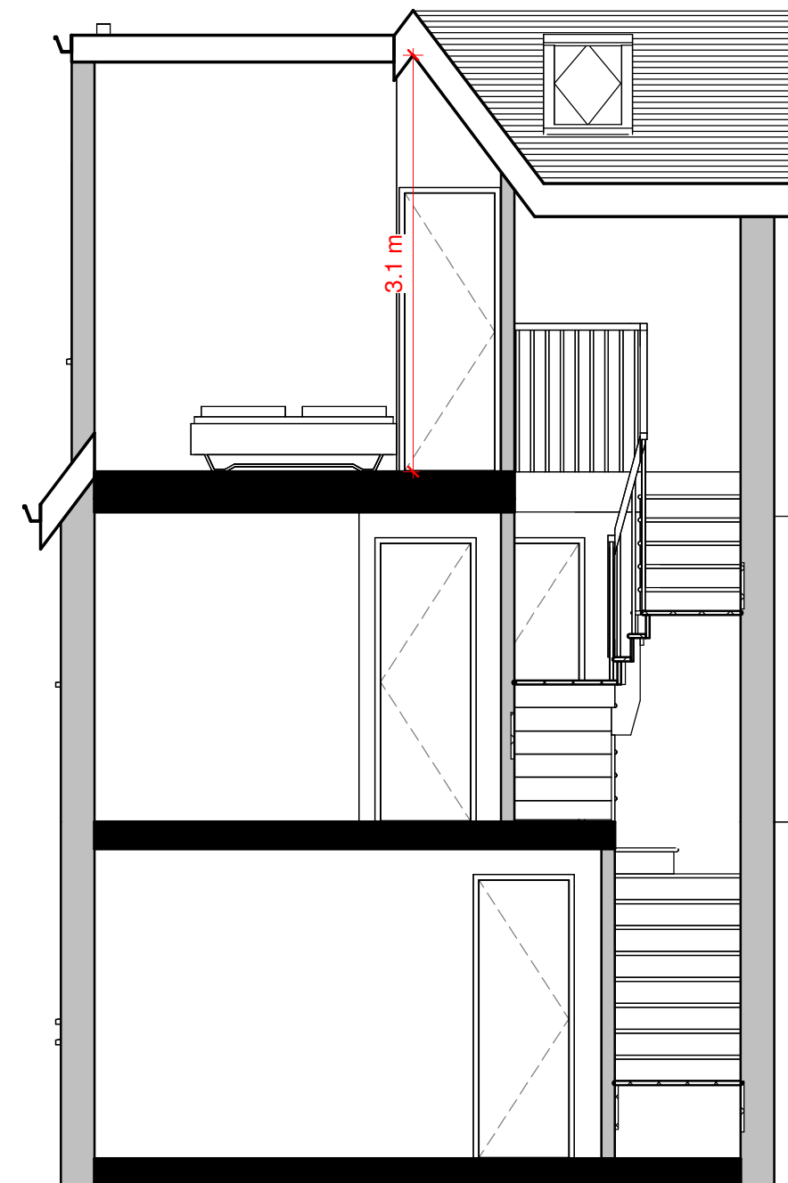
Section B-B 1 : 50
