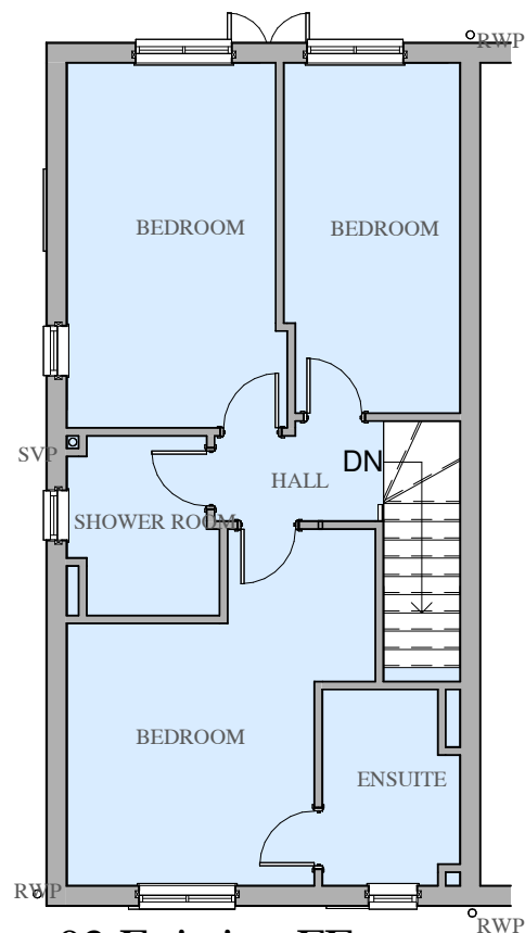
02 Existing FF 1 : 100
