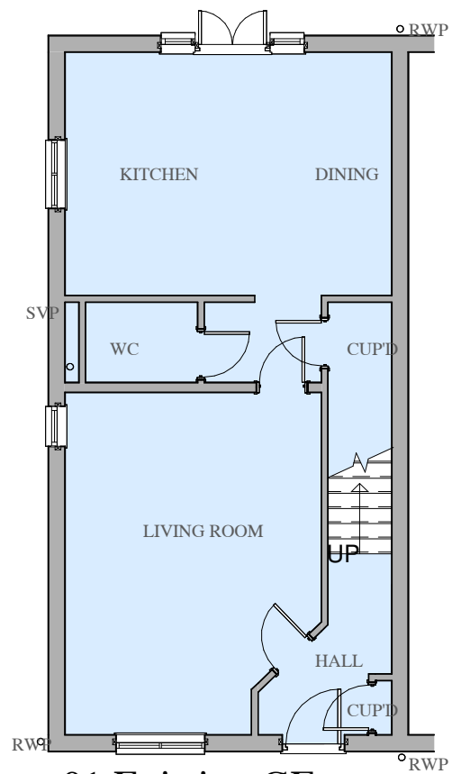
01 Existing GF 1 : 100
