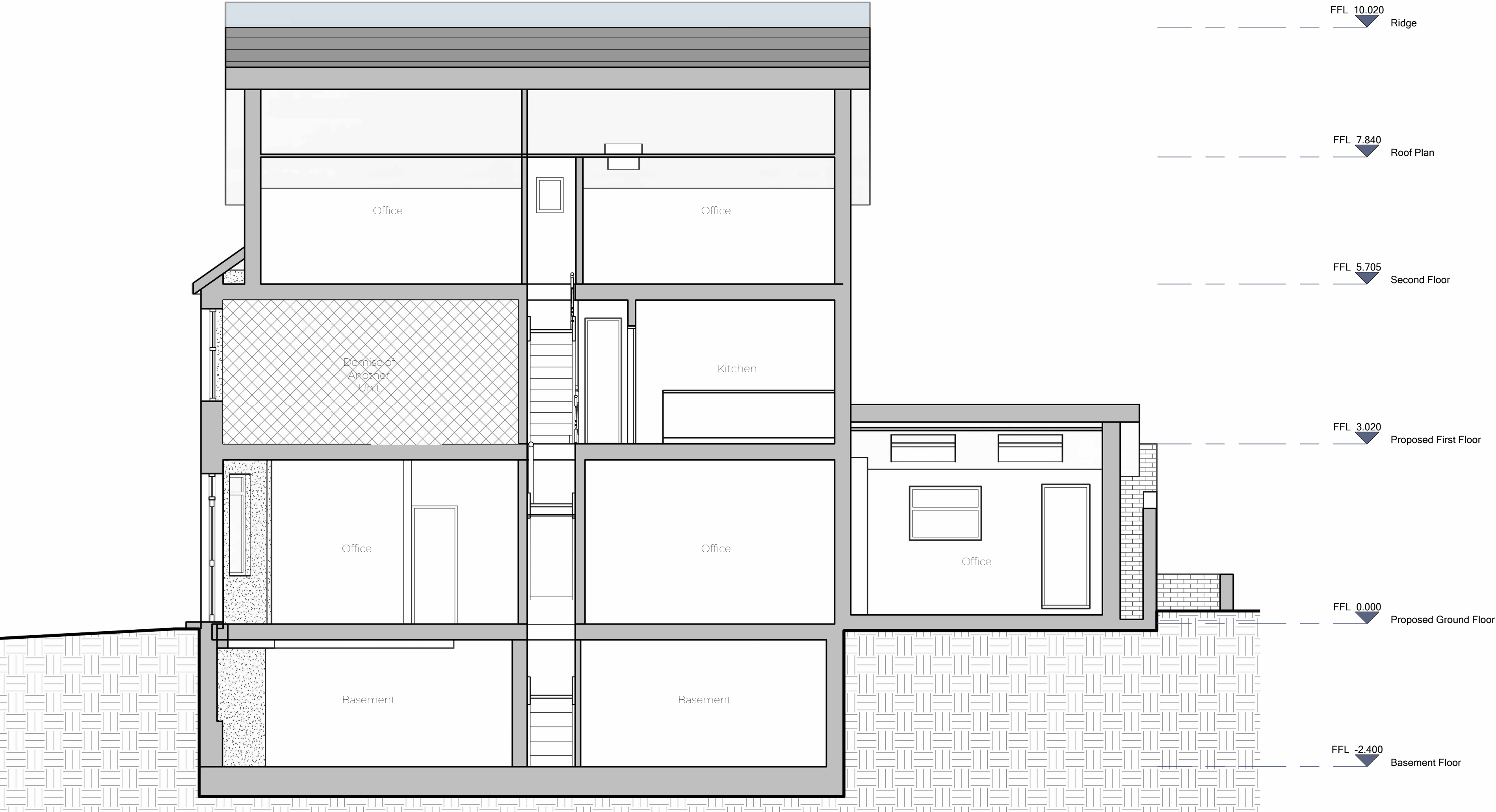
Section A-A 1 : 50
