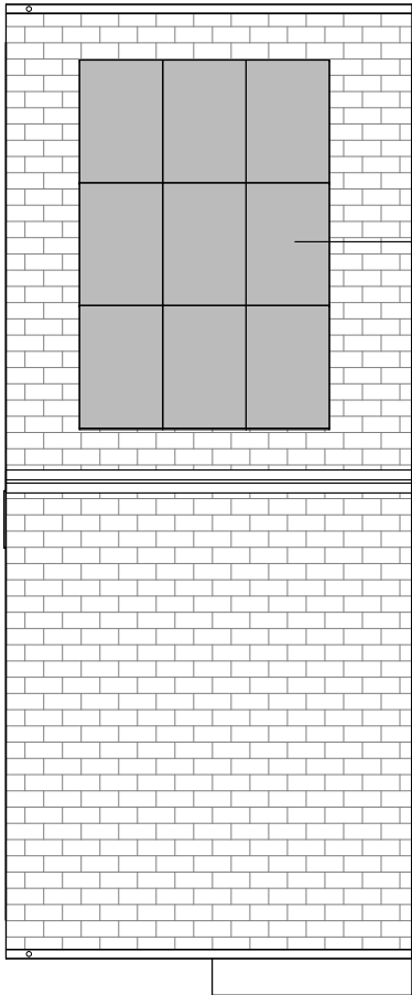
Roof Plan 1 : 100
