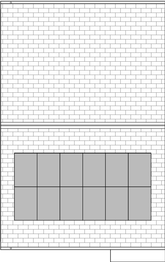
Roof Plan 1 : 100
