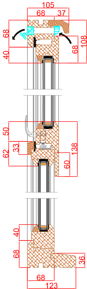
Section A-A
