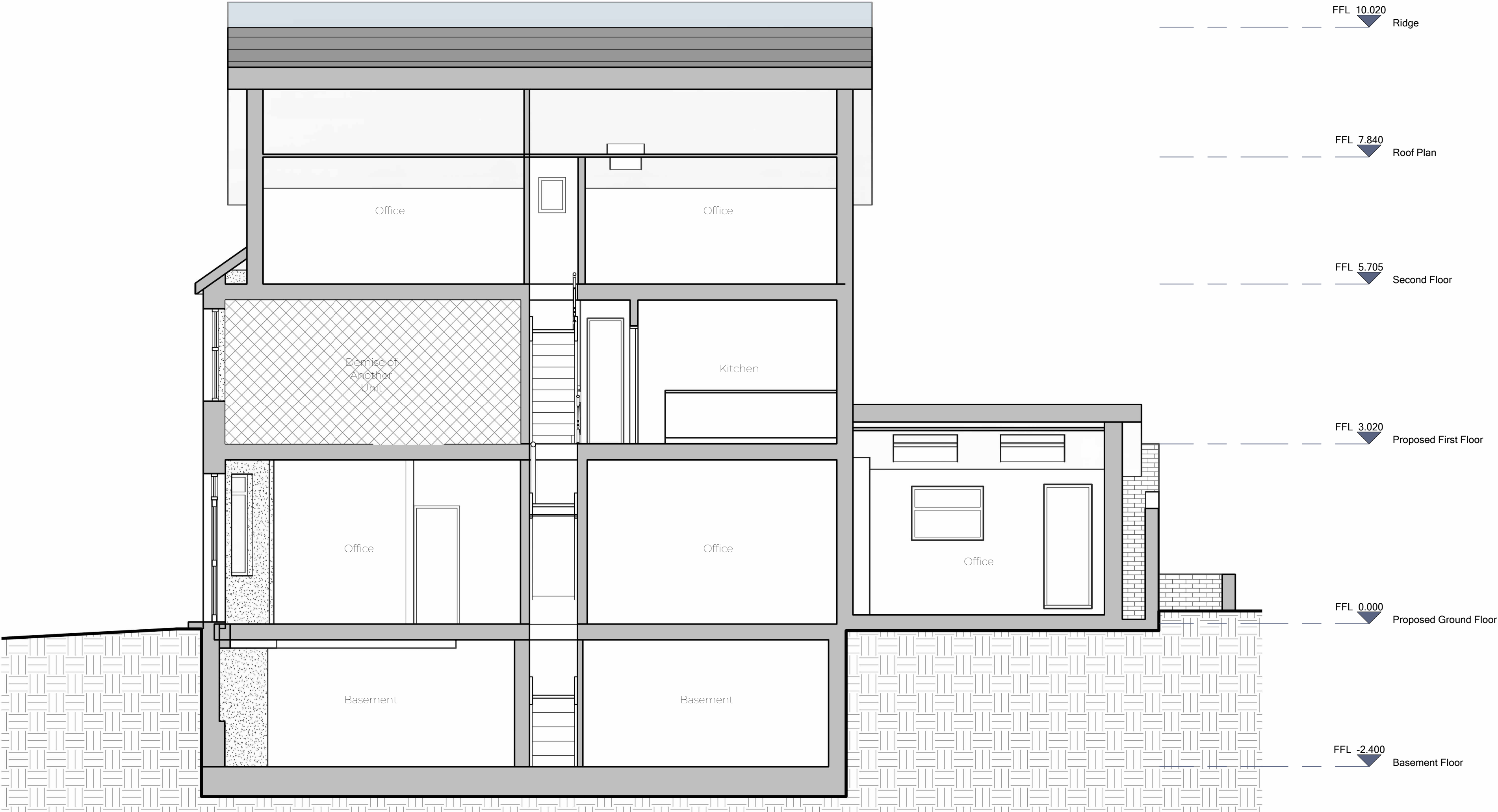
Section A-A 1 : 50
