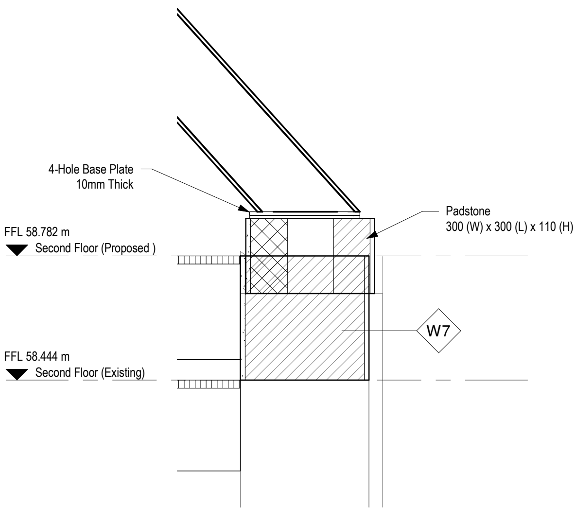
3 Section 6 - Callout 1 1 : 10
