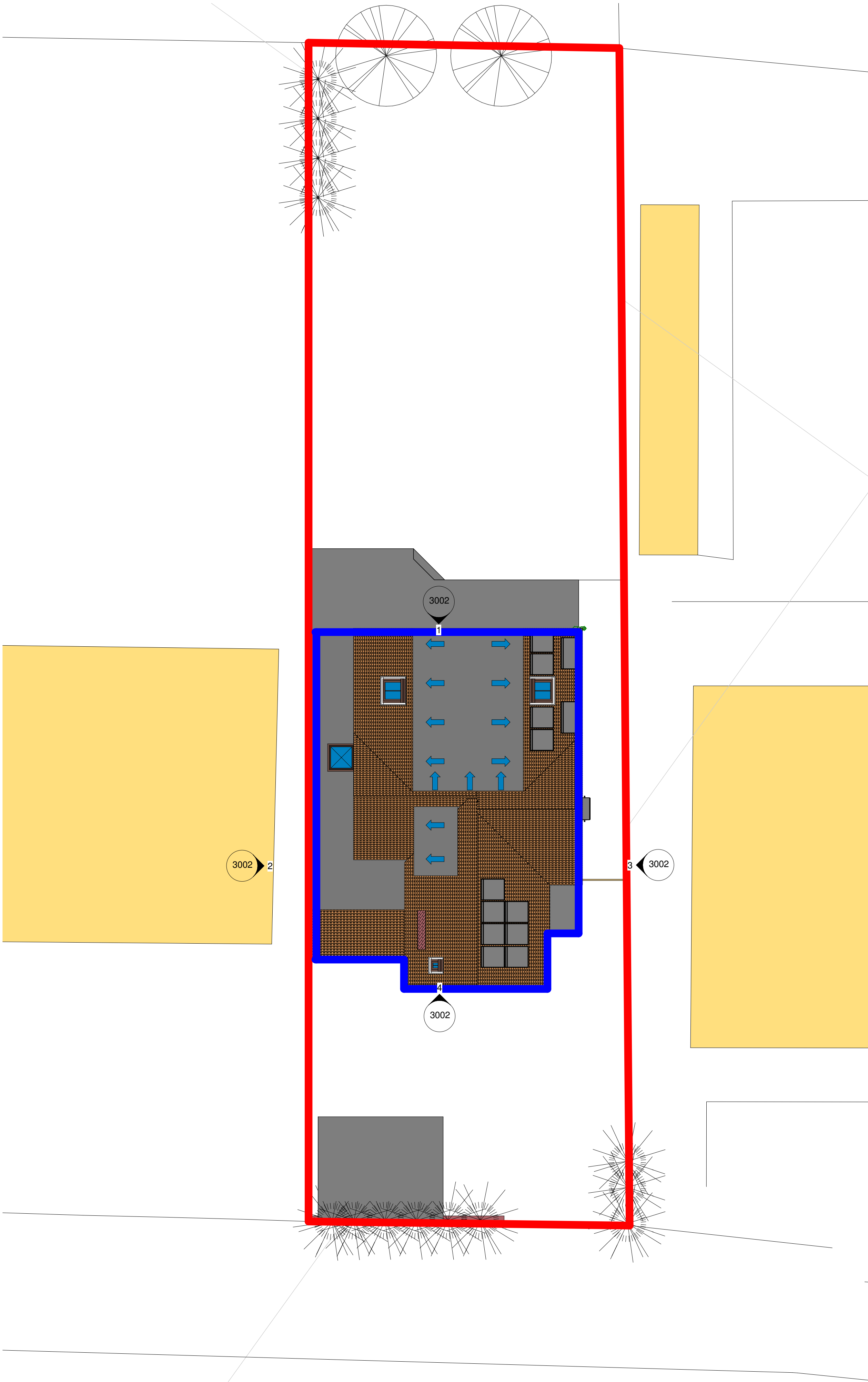
2 Site Layout (Option 1) 1 : 100
