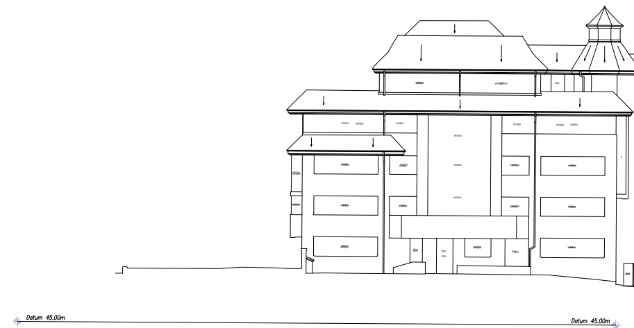
Elevation E4
