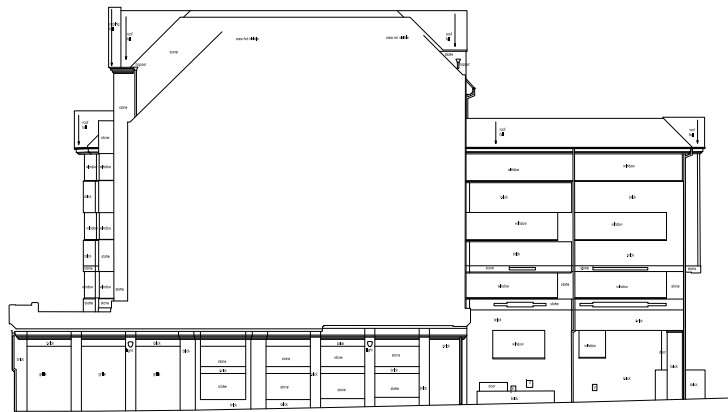
datum 45.00m datum 45.00m Elevation E8
