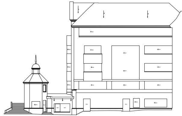
datum 45.00m datum 45.00m Elevation E6
