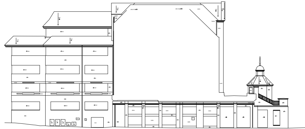
datum 45.00m datum 45.00m Elevation E7
