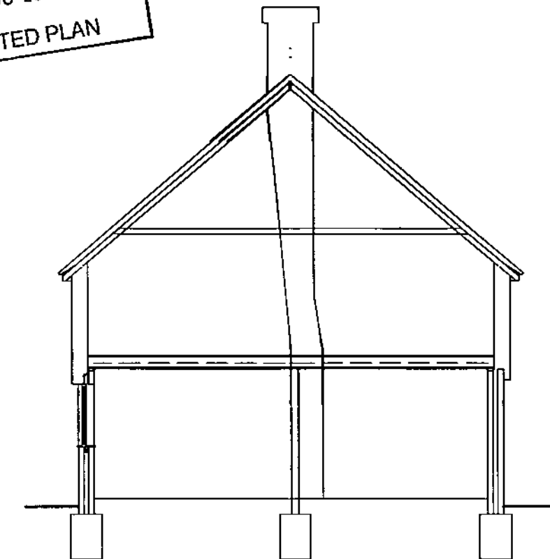
SECTION A-A 1:100
