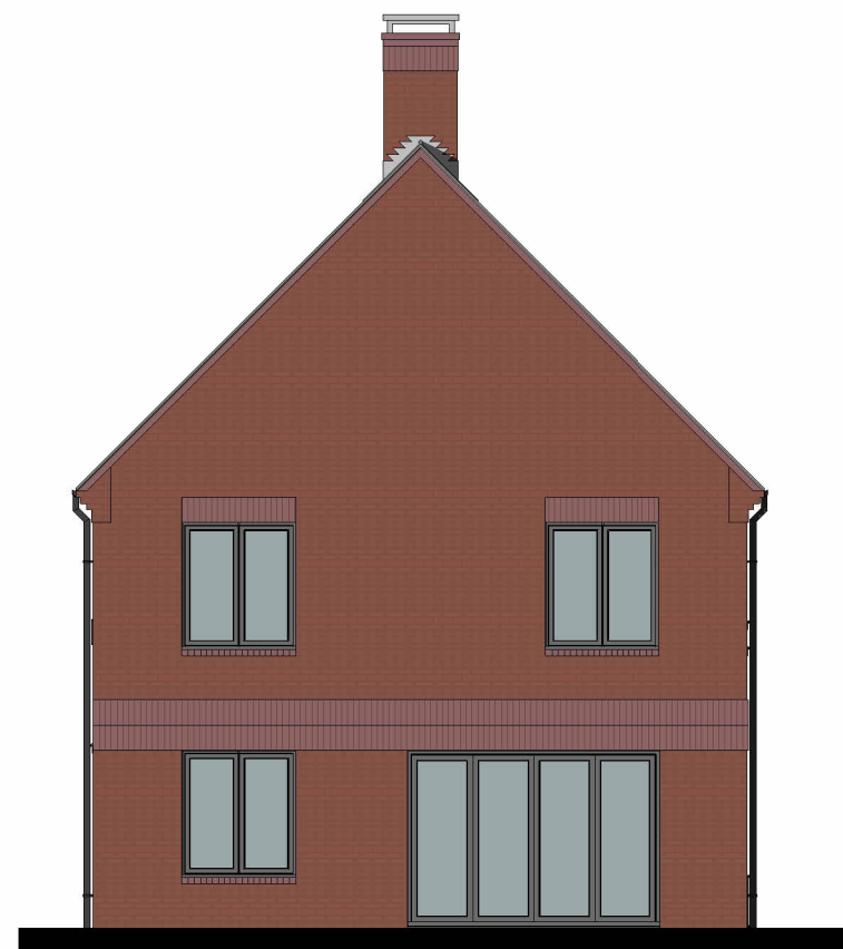
Left Flank Elevation
