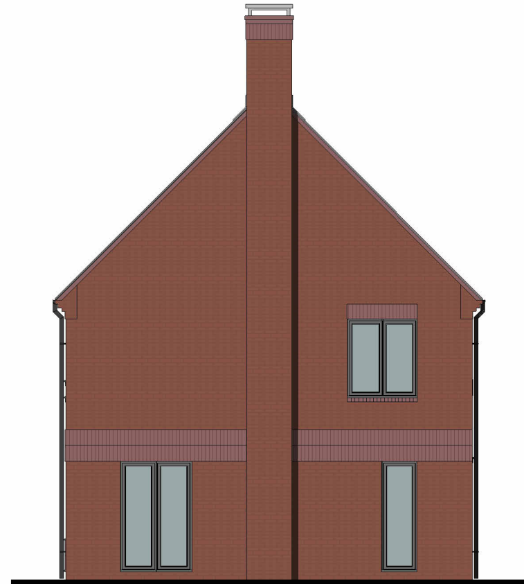
Right Flank Elevation
