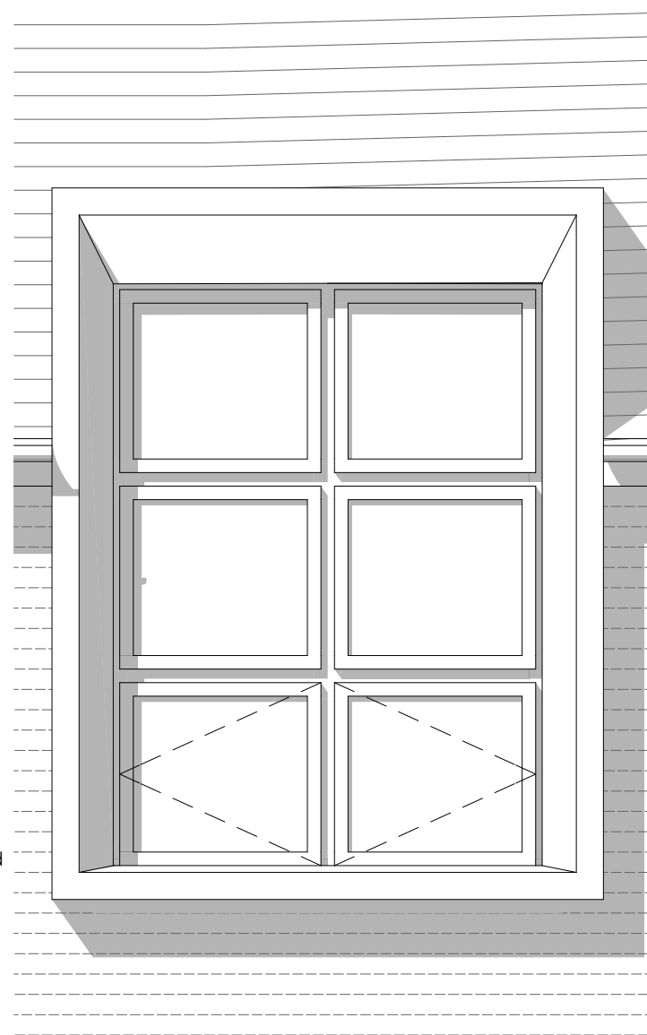
ELEVATION | 1:25 @ A3
