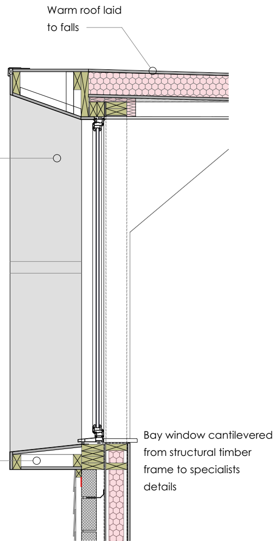
SECTION | 1:25 @ A3
