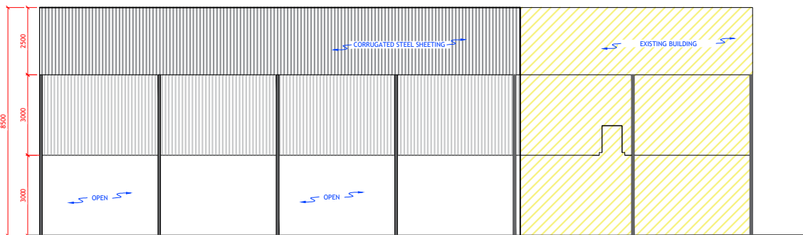
5 NORTH ELEVATION SCALE: 1:200 @ A3
