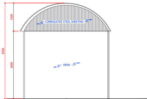
2 EAST ELEVATION SCALE: 1:200 @ A3
