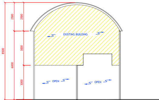
3 WEST ELEVATION SCALE: 1:200 @ A3
