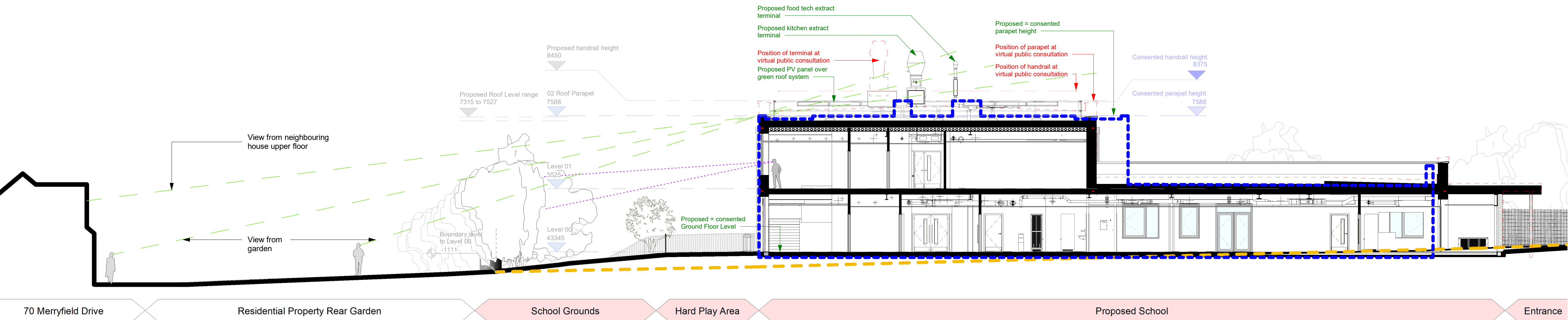
1 Site Section AA 1 : 125
