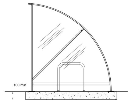
END ELEVATION
