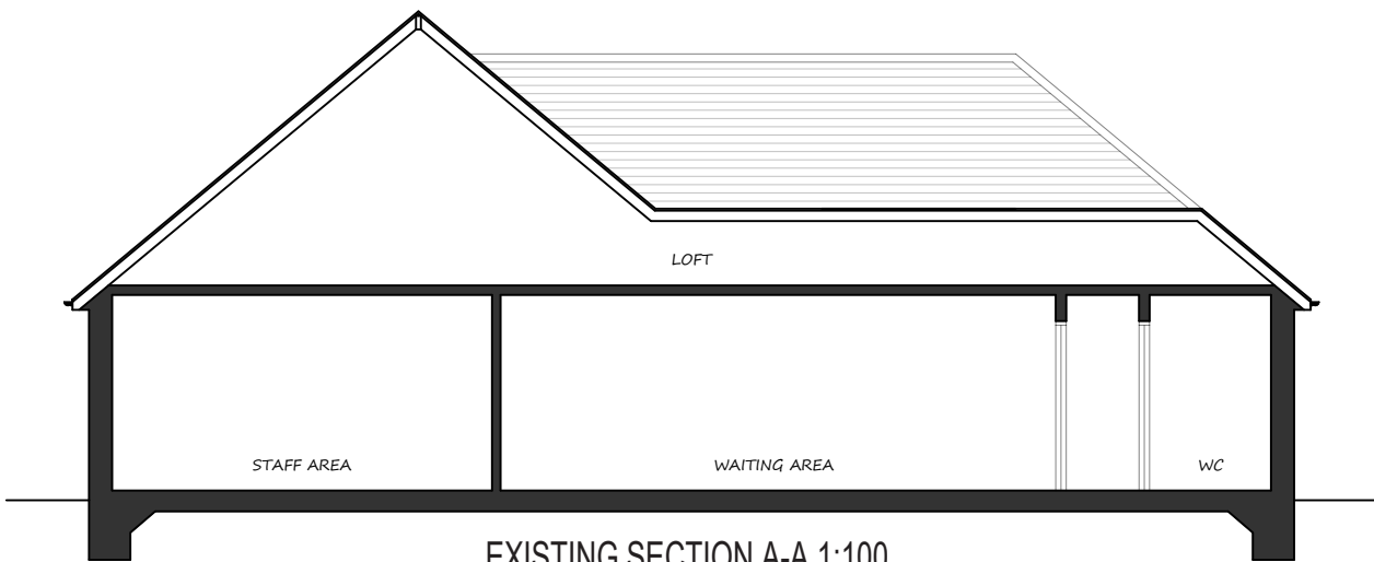
EXISTING SECTION A-A 1:100
