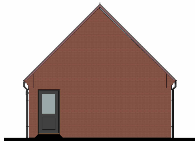
Right Flank Elevation
