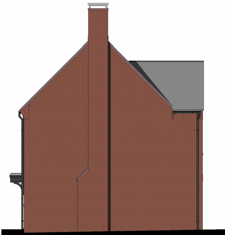
Right Flank Elevation
