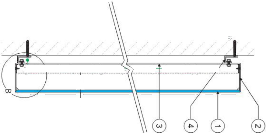
SECTION A-A 1:5
