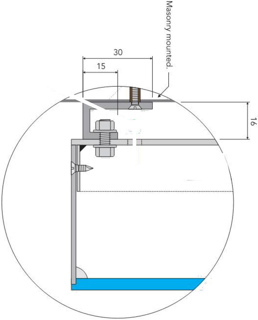
DETAIL B 1:1
