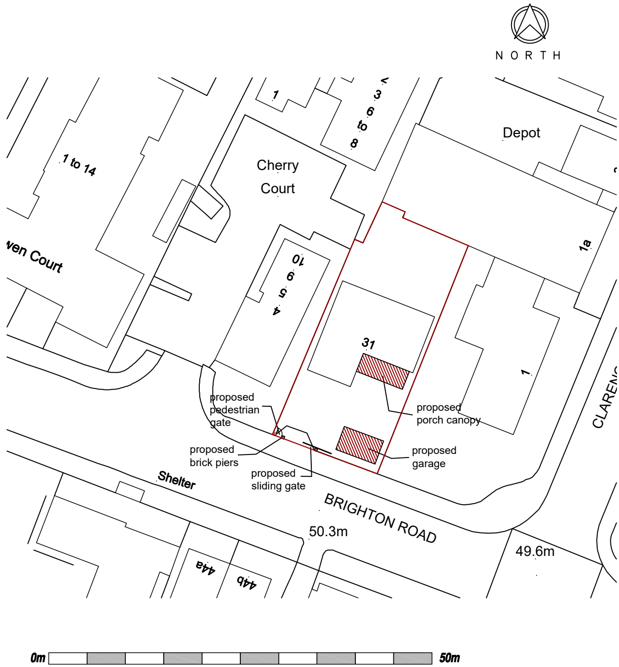
SITE/BLOCK PLAN (1:500)
