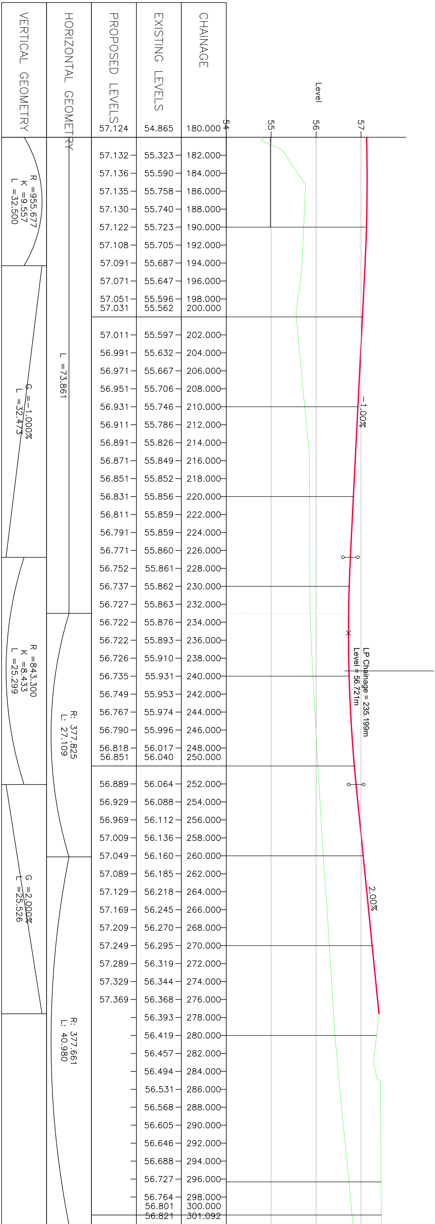
ALG - SPINE ROAD 1 - CL CH 180.000m TO 301.092m SCALE: H 1:250, V 1:50. DATUM: 54.000
