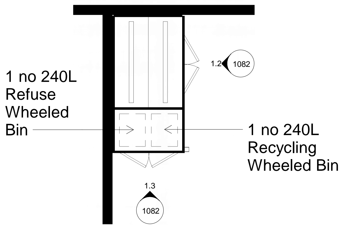
1 Type 1_Plan 1 : 50
