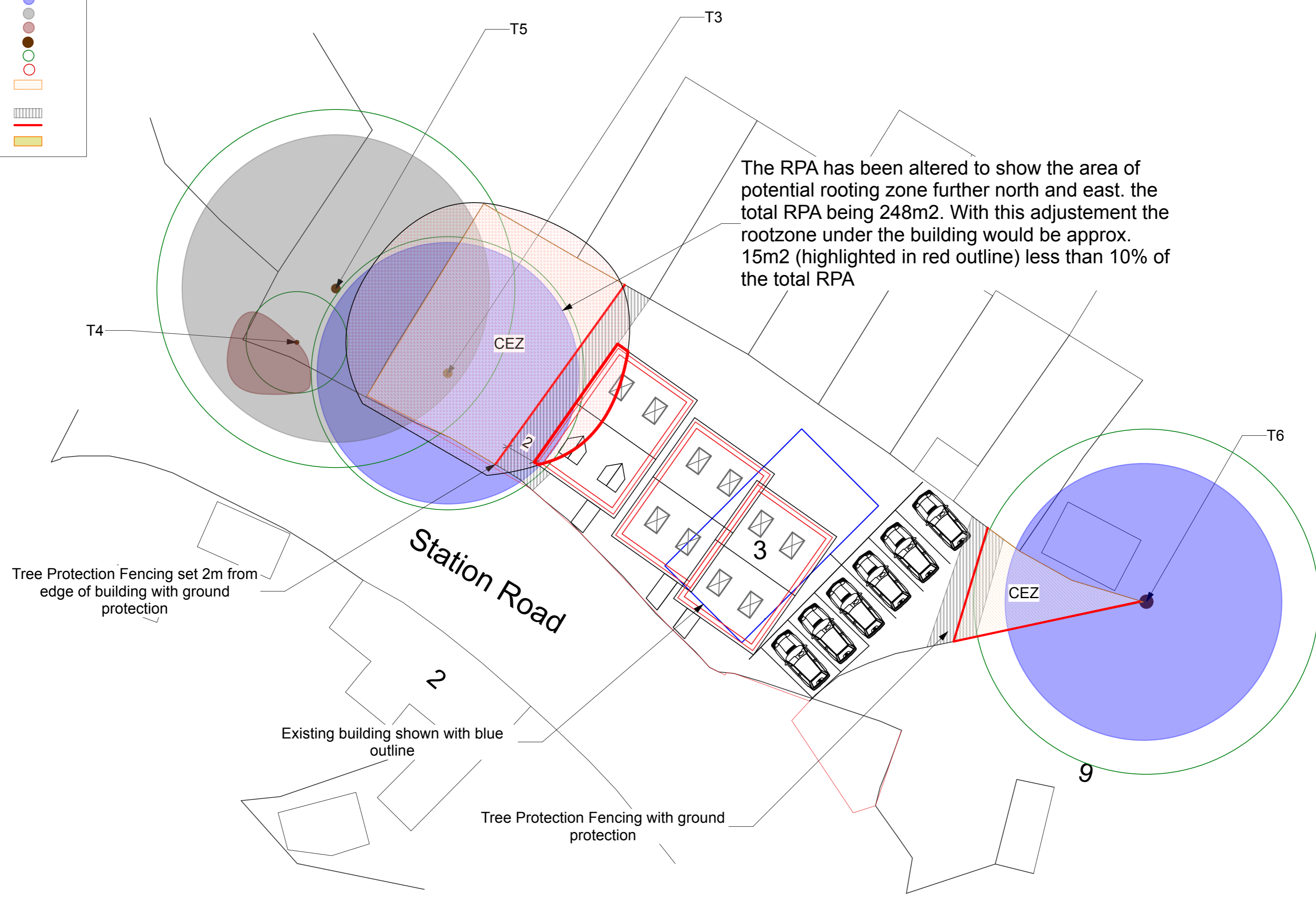
1 Tree Protection Plan Scale: 1:200
