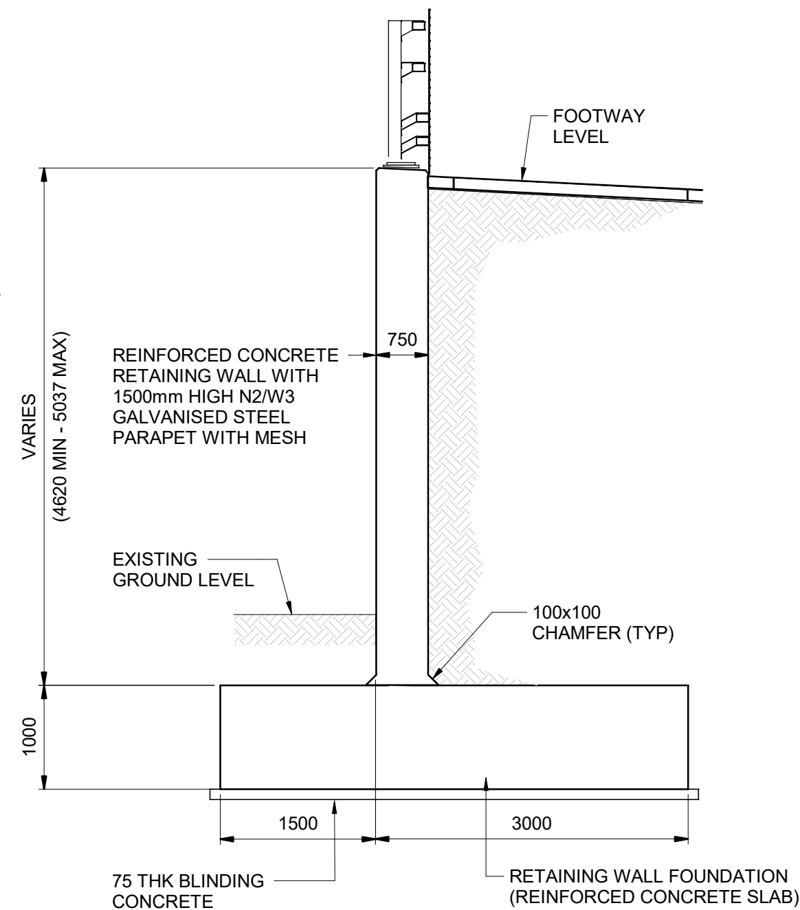
C SECTION C 00001 1 : 50
