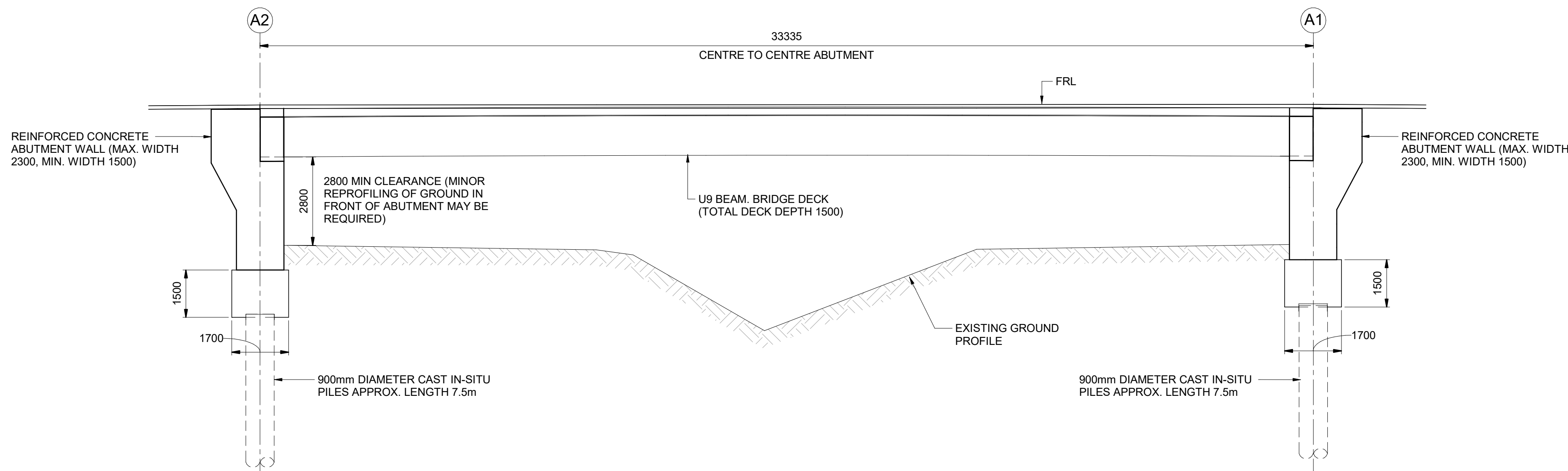
D SECTION D 00001 1 : 100
